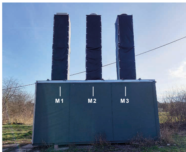
Obrázek 1: stavební buňka se třemi měřenými světlovodnými sestavami (zleva M1 SUNIZER, M2 SOLATUBE, M3 SUN LINE ONE)
